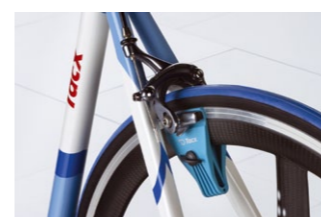
◀ 7511 74580 Fékpofa-beállító
